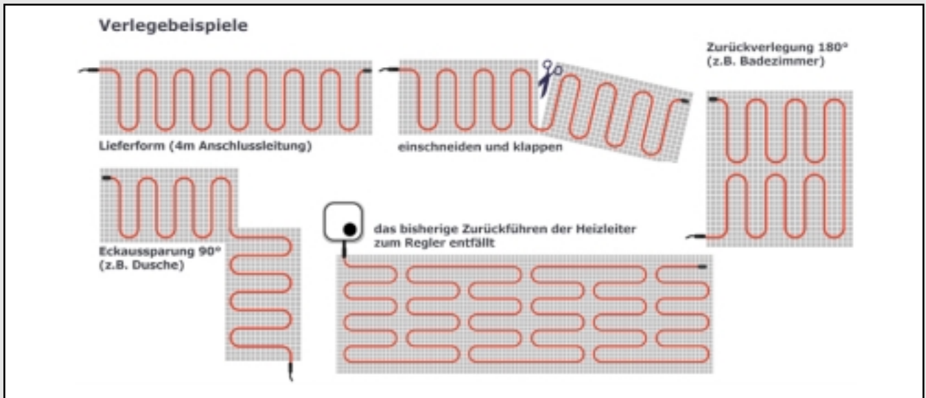
Verlegebeispiele
