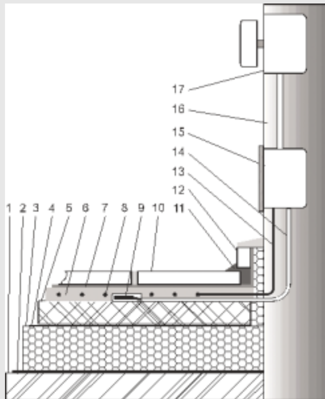
Funktionsaufbau Bodentemperierung
