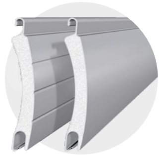
Aluminiumprofil A44 optional in glatter Optik
