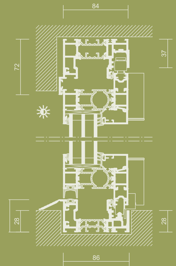
Vertikalschnitt | o.M.
