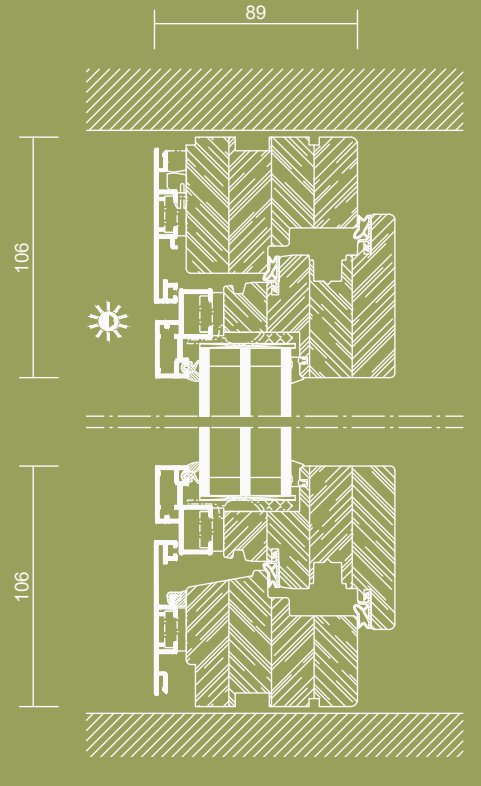
Flächenbündig
