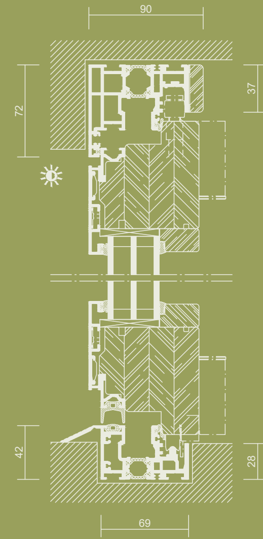
Vertikalschnitt | o.M.
