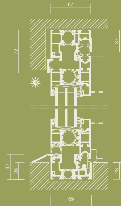
Vertikalschnitt | o.M.
