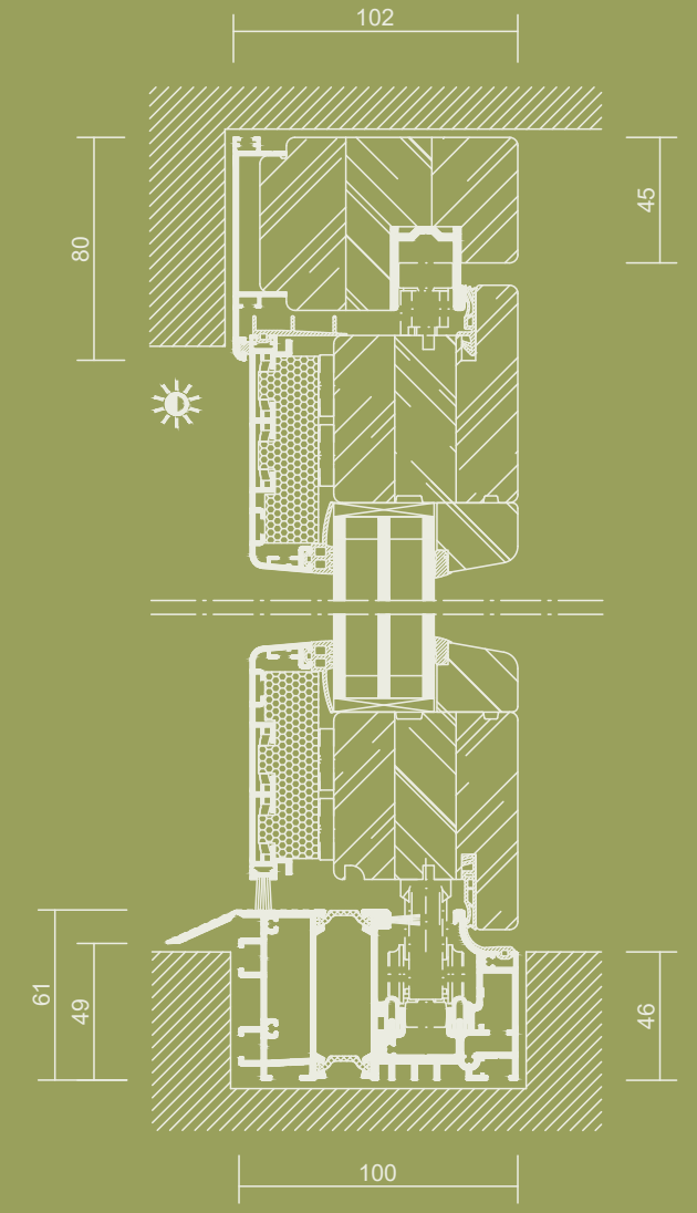
Vertikalschnitt | o.M.
