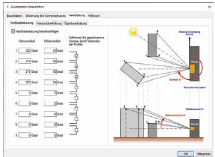
Importierte Revit-Daten zum Berechnen einer Fremdbeschattung, z. B. Nachbarbebauung.
