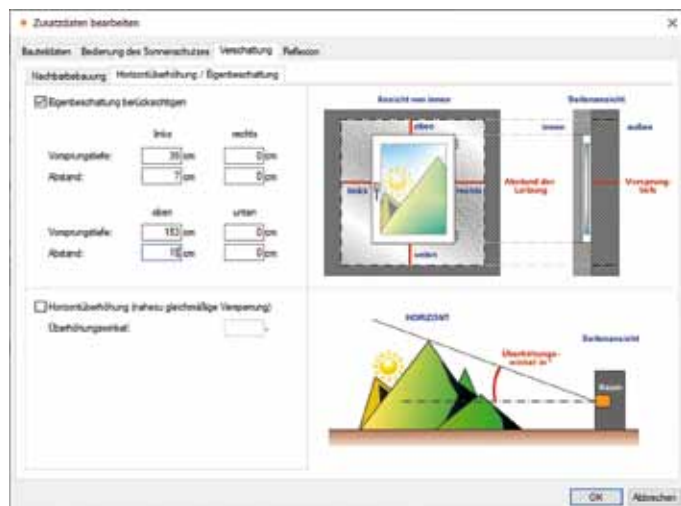
Aus Revit in die SOLAR-COMPUTER-Simulations-Programme importierte Daten zum Berechnen der Eigenbeschattung.
