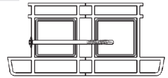
SPC4 ohne Vorbohren der letzten Kammer
