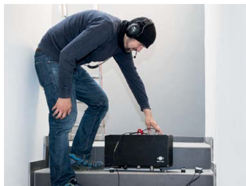
Schallmessung
