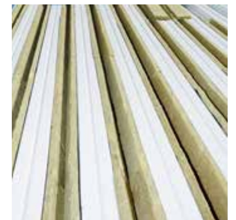
Einlegen von Akustik-Profilfüllern in Trapezprofile
