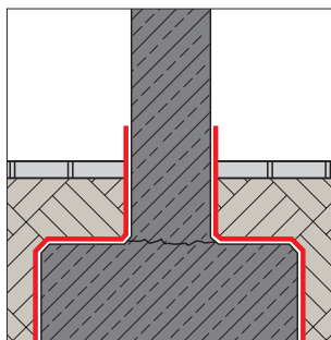
Abdichtung von Stützen-Fundamenten
