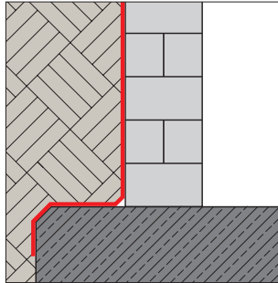
Erdberührte Außenabdichtung
