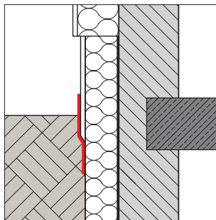
Putzabdichtung
