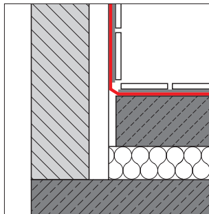
Fliesen- & Platten-Verbundabdichtung
