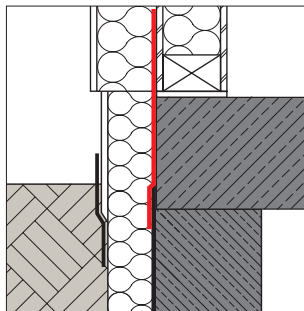
Sockelabdichtung im Holzrahmenbau
