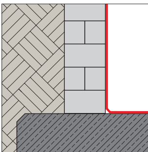
Nachträgliche Innenabdichtung
