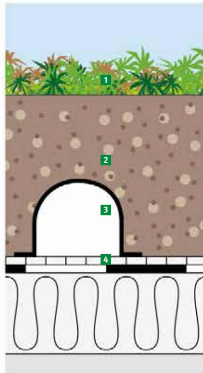
1 Vegetation 2 Extensiv-Einschichtsubstrat M 3 Triangel-Wasserleitprofil WLP Plus 4 Trenn-, Schutz- und Speichervlies RMS 300
