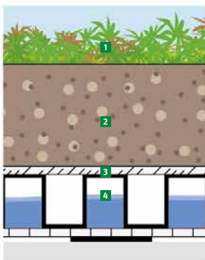
1 Vegetation 2 Extensiv-Substrat E 3 Filtervlies FIL 105 4 Drän- und Wasserspeicherelement FKD 25 bis 1,5 cm stehendes Wasser
