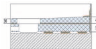
waagerechter Ablauf mit Unterbauelement
