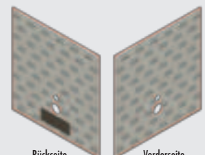
Rückseite Vorderseite TEC-VWD-PV – 1250 x 1200 x 20 mm
