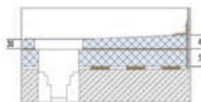
senkrechter Ablauf mit Unterbauelement
