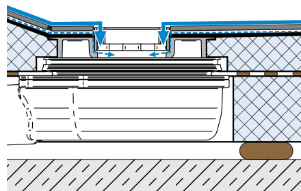
Abb. 2 – LUX ELEMENTS®-TUB-LINE, Linienentwässerung
