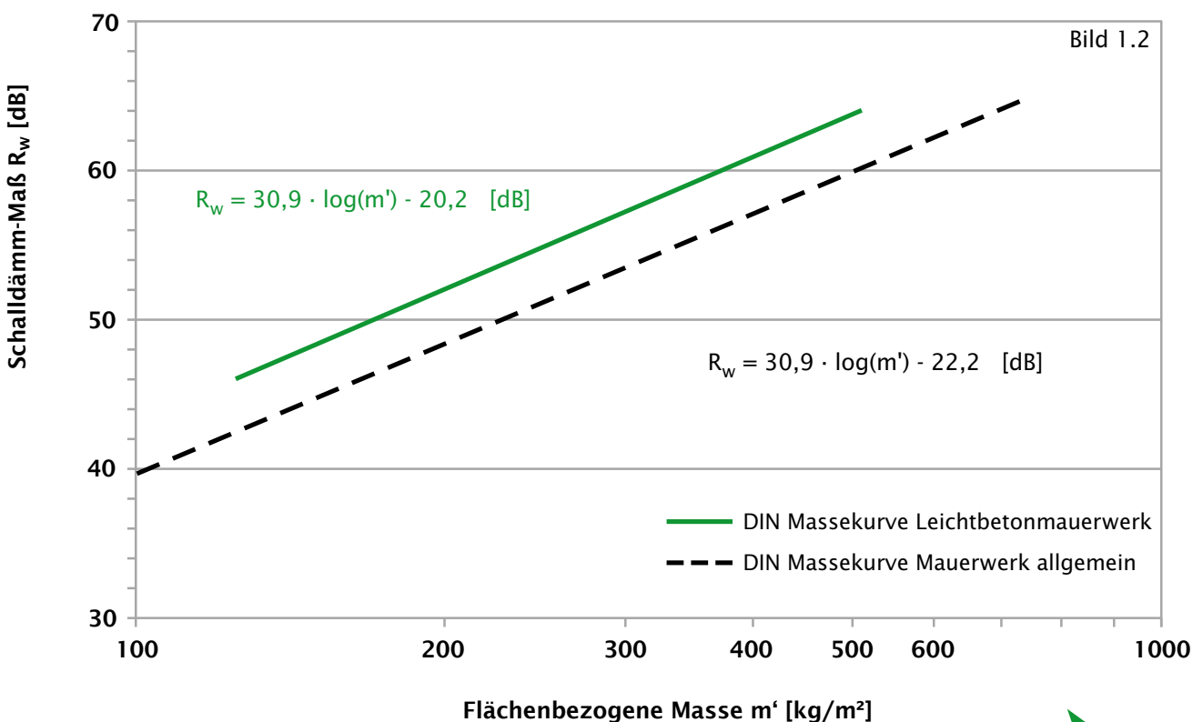
Bild 1.2: Schalldämmung von Leichtbetonmauerwerk in Abhängigkeit der flächenbezogenen Masse. Im Bereich von m' 140\text{--}480 \text{ kg/m}^2 ist das Schalldämm-Maß R_w um 2 dB höher als von Mauerwerk allgemein.
