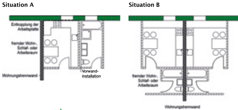
Bild 1.3: Günstige Position von Installationen gleichartiger Räume an einer Innenwand und einer Wohnungstrennwand [5].
