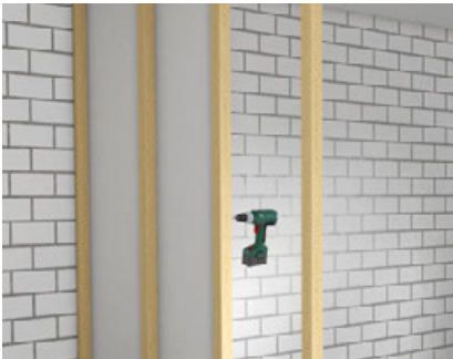
fermacell® Gipsfaser-Platten mit der fermacell Schnellbauschraube 3,9 x 30 mm (Abstand max. 250 mm) verschrauben. Senkrechte Plattenstöße erfolgen immer auf dem Holzständerwerk.
