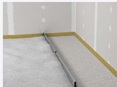
fermacell™ Wabenschüttung einbringen und abziehen
