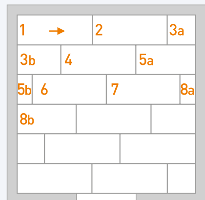
Verlegeschema 1 – Verlegung zur Tür
