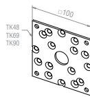
13 109.2902 Adapterplatte Teilkreis 48, 60, 90 mm, ohne Motorlager und Schrauben
