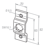
13 106.3501 Motorlager 16 x 16 mm Teilkreis 60 mm, gekröpft
