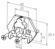
23 374.6801 für Typ 9-Vorbau-elemente- motorlager (bis 50 Nm) (vergrößert das Seitenab- zugsmaß um ca. 11 mm)
