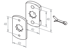
23 109.0001 Motorlager flach 16 x 16 mm Teilkreis Ø 48 mm mit Kunststoff-Distanzplatte und Splint (enthält Nr. 13 103.3901 und 13 110.5601)
