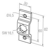
13 106.3501 16 x 16 mm Teilkreis 60 mm, gekröpft
