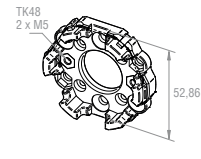
23 003.0401 Teilkreis 48mm mit Muttern 2 x M5, Teilkreis 60 mm
