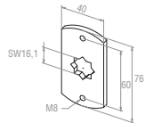
13 103.4001 Motorlager 16 x 16 mm Teilkreis 60 mm, flach
