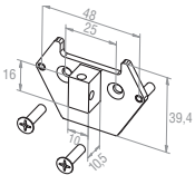
23 374.1401 10 x 16 mm, Zapfen kurz 10,5 mm (bis 50 Nm)
