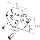
23 374.1501 10 x 16 mm, Zapfen lang 17 mm (bis 50 Nm)
