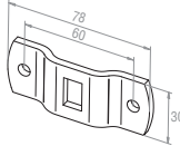
13 106.1701 Wandanker gekröpft, Teilkreis 60 mm
