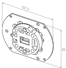
23 276.0001 Montageplatte mit Motorlager (Thyssen, Schüco, Veka, Home)
