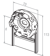
23 615.9401 für Vorbauelemente Gr. 165 mm, d = 78,2 – 79,7 mm, bis max. 30 Nm
