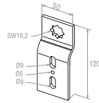
13 301.0801 Motorlager 16 x 16 mm stehend Stern
