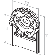
23 615.8401 für Vorbauelemente Gr. 165 mm, d = 78,2 – 79,7 mm, bis max. 30 Nm
