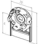
23 615.9301 für Vorbauelemente Gr. 150 mm, d = 70,7 mm, bis max. 30 Nm
