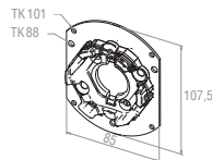
23 615.7101 Montageplatte mit Kunst- stofflager bis max. 30 Nm (Thyssen, Schüco, Veka, Home)
