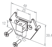
23 374.3301 Adapterplatte, 12 x 12 mm, Höhe 12 mm, bis 50 Nm
