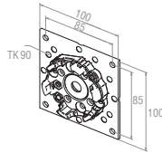
23 615.9901 Grundplatte mit Motorlager z. B. für VEKA- Variant-Elemente
