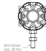
23 615.3501 Spezial Bolzenlager mit Höhenverstellung über M10 Bolzen, max 80 Nm
