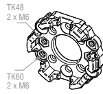
23 003.0101 Teilkreis 48/ Teilkreis 60 (Alu) mit Muttern 4 x M6
