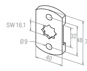
13 110.5601 Distanzplatte für 13 103.3901 (nicht als Lager einsetzbar)
