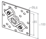
23 833.0001 Grundplatte mit Motorlager 16 x 16 mm Teilkreis 48, 60, 90 mm
