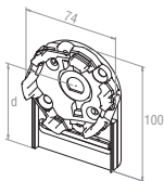
23 615.9201 für Vorbauelemente Gr. 137 mm, d = 64 – 65,5 mm, bis max. 30 Nm
