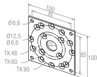
13 109.2902 Grundplatte mit Teilkreis 48/60/90 mm (ohne Motorlager und Schrauben)
