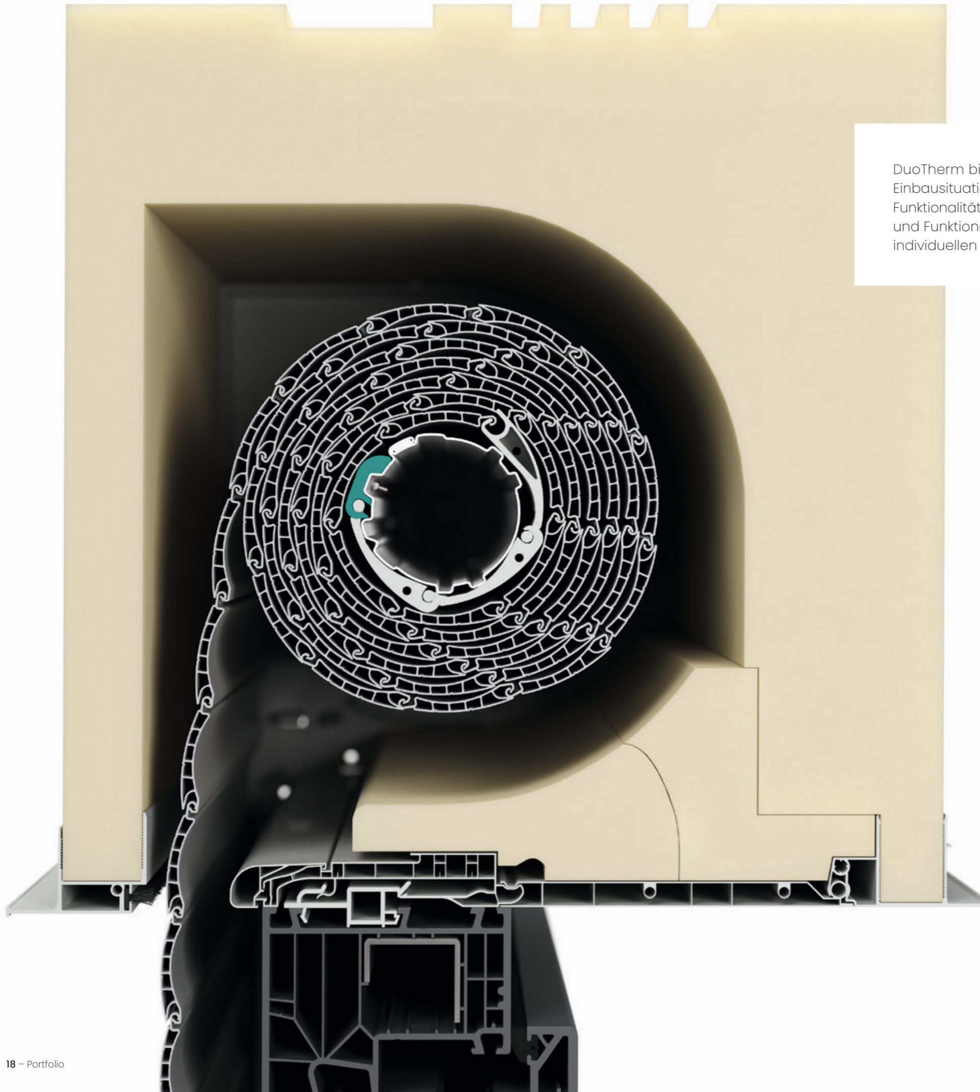
Neubauaufsatzkästen
