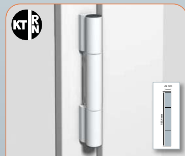
Rollenband für Kunststofftüren Paumelle cylindrique pour portes PVC Butt hinge for PVC doors
