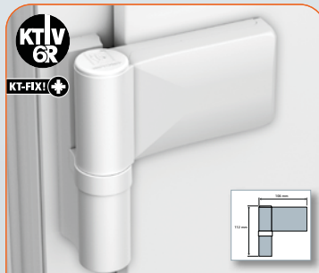
Für repräsentative Eingangstüren Pour portes d'entrée haut de gamme For representative door entrances
