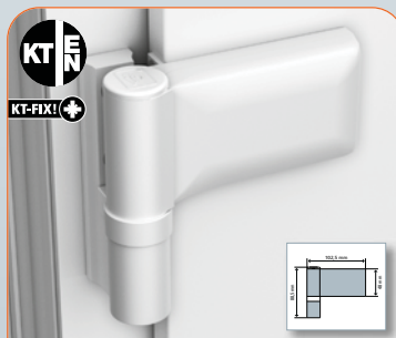
Für Haus- und Nebeneingangstüren Pour portes d'entrée principales et secondaires For residential and side entrance doors
