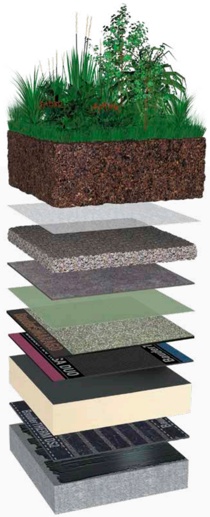
Schüttstoff-Dränage mit BauderGREEN MD BS Mineraldrän
