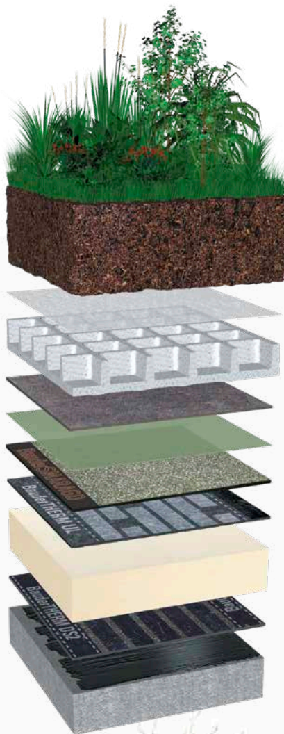
Hohes Speichervermögen mit der BauderGREEN WSP 75 Wasserspeicherplatte
