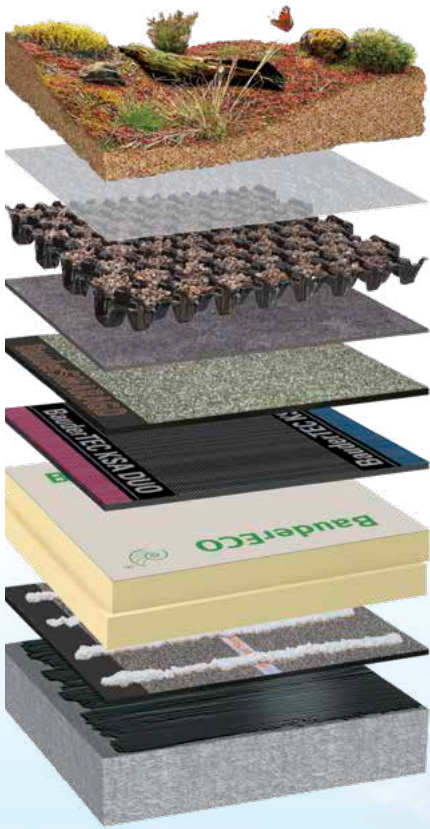
Wasserrückhalt mit dem BauderGREEN RE 40 Retentionselement
