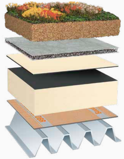
Preiswerte Dachbegrünung mit der BauderGREEN SDF-Matte
