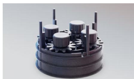
Terrassen-Stelzlager
