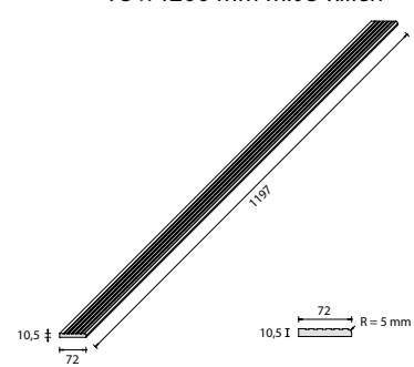
Treppenkante 75 x 1200 mm mit 5 Rillen
