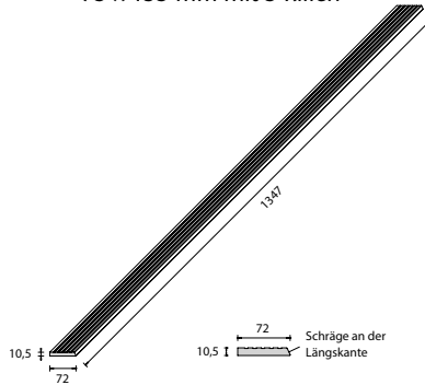
Treppenkante mit Schräge 75 x 135 mm mit 5 Rillen
